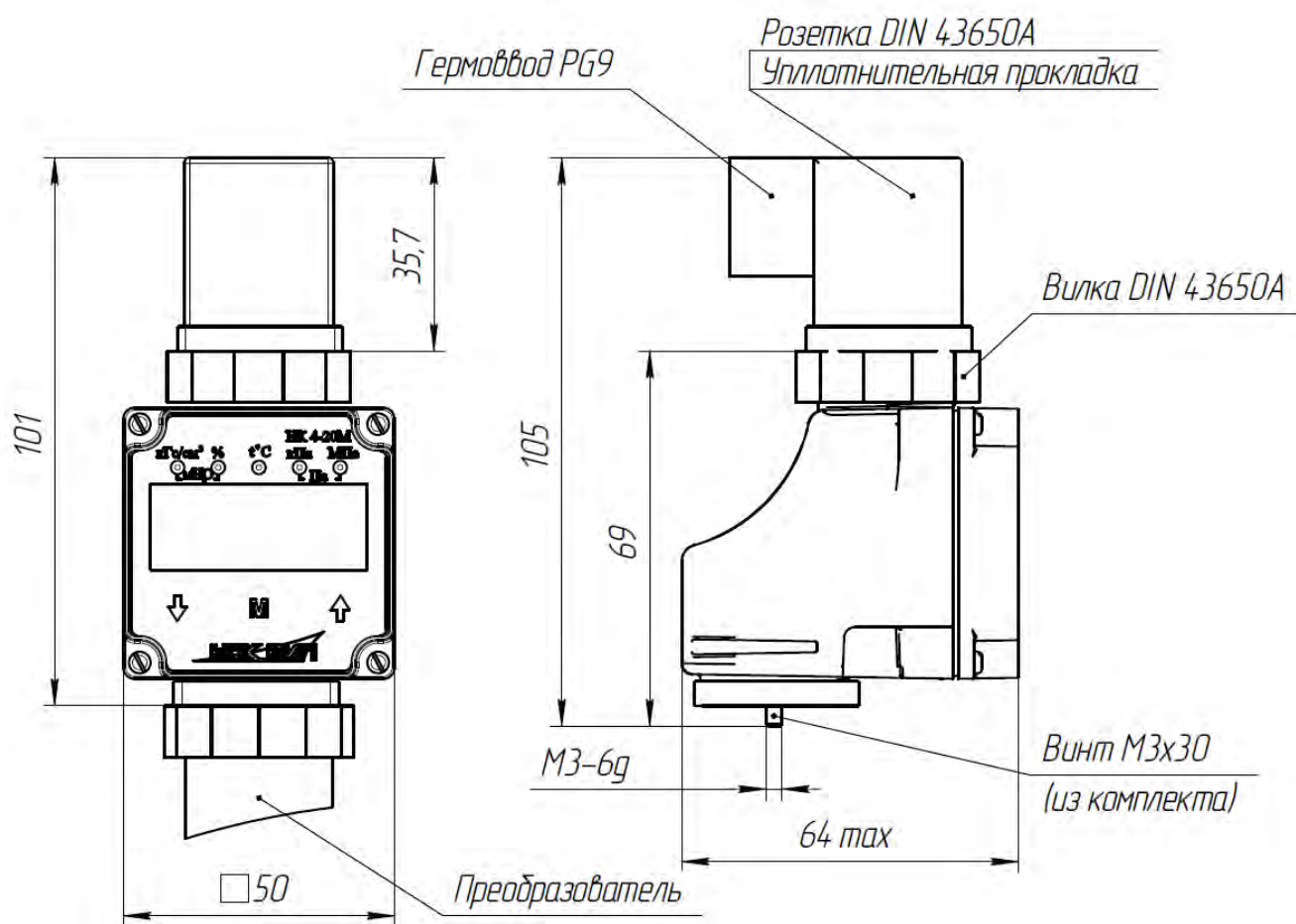
Рисунок Г.1 Габаритно-присоединительные размеры ИК 4-20М
